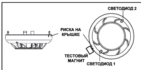
Рис. 3: Тестирование магнитом
