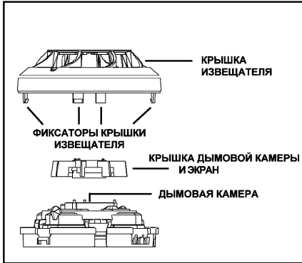
Рис.2: Обслуживание извещателя
